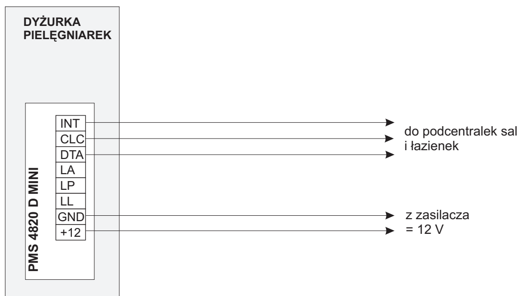
Sposób podłączenia matrycy PMS 4820 D do instalacji przyzywowej
